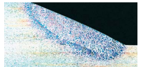
Metalurgia através dos gases de processo: controlo da proporção austenite-ferrite na soldadura TIG de aço duplex com VARIGON® N
