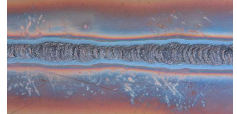
Cordão TIG, lado da raiz, nenhuma protecção da raiz
