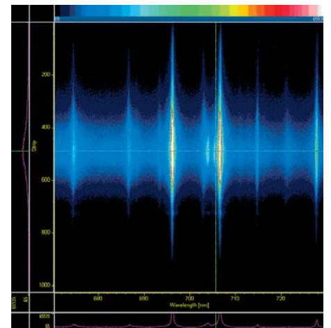
Utilização de métodos científicos para investigar o plasma - processos físicos no arco: secção de uma análise espectral no processo de soldadura MIGp de alumínio com VARIGON® He30S
